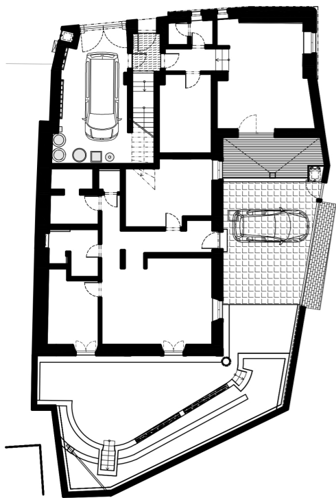
Půdorys 1.NP
