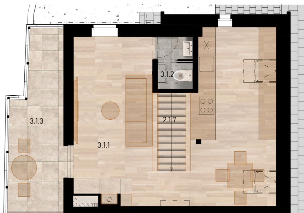
Půdorys Podkroví
